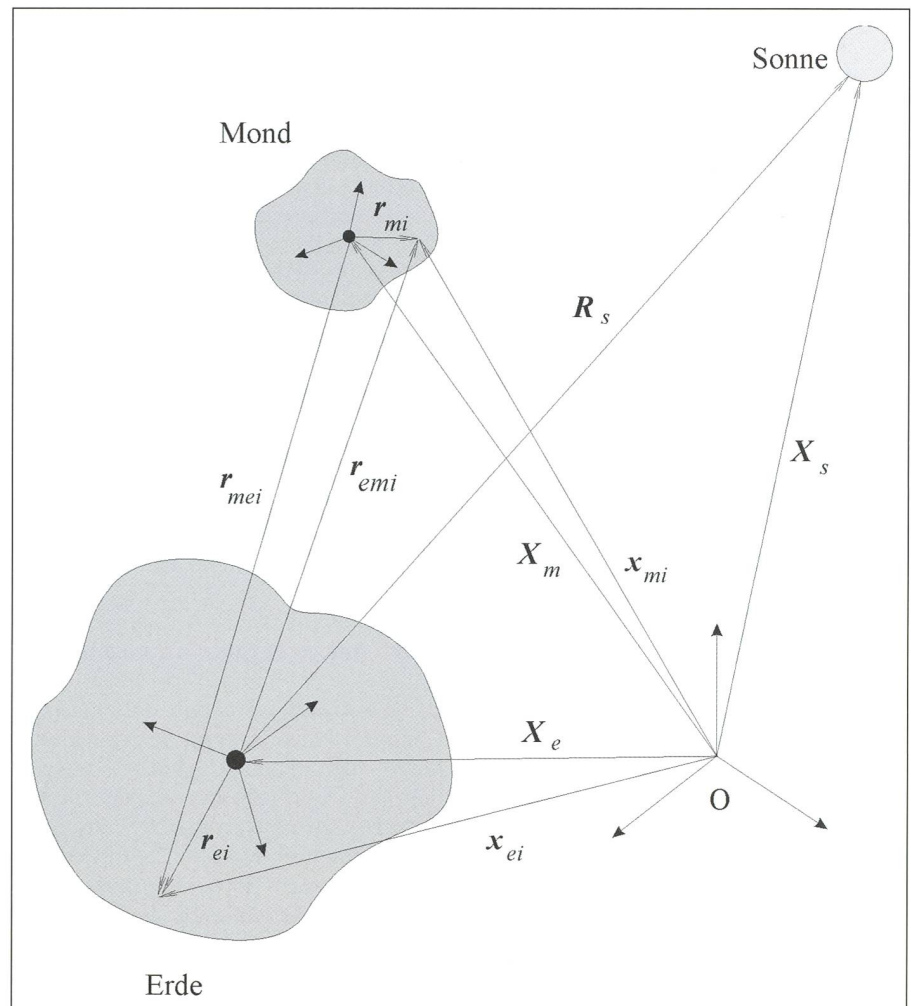
Fig. 11: Das Dreikörperproblem Sonne-Erde-Mond.
