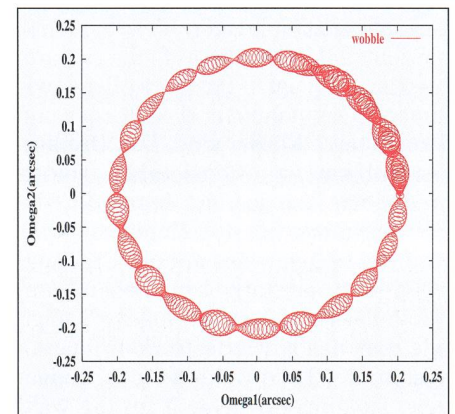
Fig. 13: Die Polschwankung während eines Jahres.
