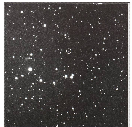
Fig. 4: Zimmerwalder CCD-Aufnahme des NEO 2001WA25 vom 4. Januar 2002. Der Kleinplanet ist das schwache Objekt im weissen Kreis ( m_v \sim 18.5 ; Ausschnitt circa 12 \times 12 Bogenminuten).
