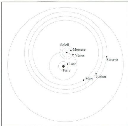
Figure 15: modèle de Tycho Brahé.
