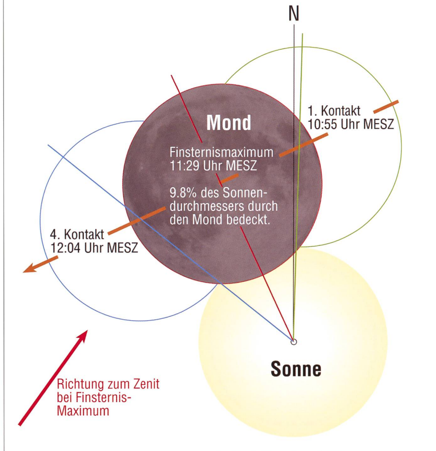
Figur 7: Sonnenfinsternis vom 1. August 2008, Verlauf für einen Beobachter in Schwarzenburg. 1. Kontakt (grün), Finsternismitte (rot) und 4. Kontakt (blau). Die Bahn des Mondzentrums (braun) in Bezug auf die Sonne zeigt, dass der Mond abgehend ist, das heisst die Finsternis findet in der Nähe des absteigenden Knotens statt. (Grafik nach E. Laager: Thomas Baer)
