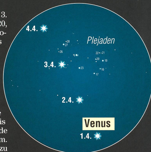
Abbildung 1: Venus passiert die Plejaden. (Grafik: Thomas Baer)
