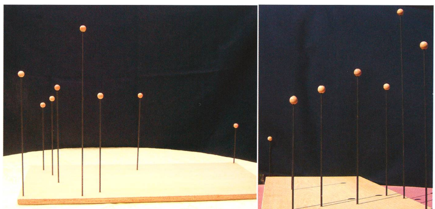
Abbildungen 3 und 4: In einem Sperrholzbrett stecken Stäbe, die oben eine Kugel tragen. Diese zeigen die räumliche Verteilung der hellen Sterne eines zunächst unbekannten Sternbildes. Dem Betrachter hat man verraten, wo im Modell unsere Sonne wäre. Schaut man von diesem Ort her (Bild rechts), erscheint das vertraute Bild des Himmelswagens. Das «Reiterchen» Alcor steht weit hinter Mizar, oberhalb diesem knapp sichtbar. (Bilder: Erich Laager)
