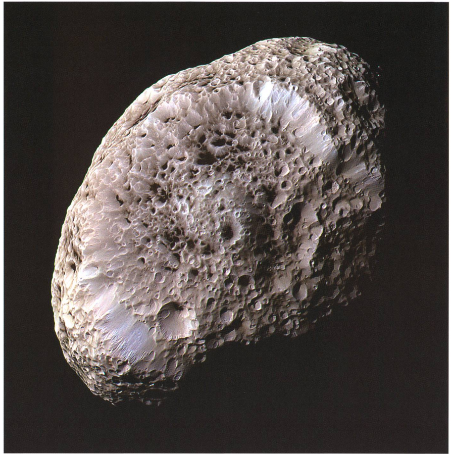
Abbildung 3: Hyperion, ein 270 km grosses Wespennest, das mit einer chaotischen Eigenrotation um Saturn taumelt. (Bild: NASA)
