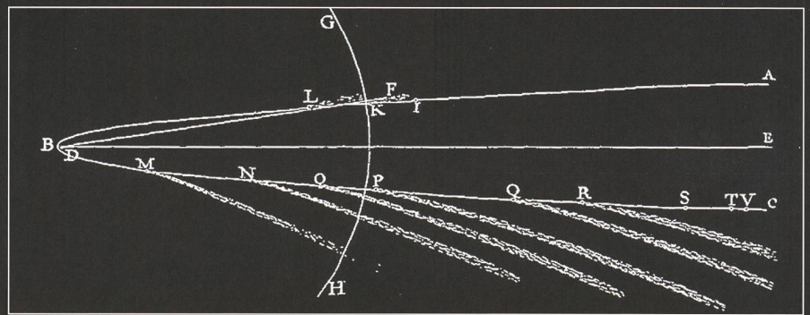
Abbildung 2: Die Bahn des Kometen Kirch (C/1680 V1) weist eine grosse Ähnlichkeit mit jener von ISON auf, was die Vermutung nahelegt, dass beide Schweifsterne womöglich einen gemeinsamen «Mutterkometen» hatten. Kirch gilt aber als langperiodischer Komet mit einer Umlaufzeit von 9356 Jahren. Bei ISON vermutet man indessen eine hyperbolische Bahn. (Zeichnung: Sir Isaac Newton)
