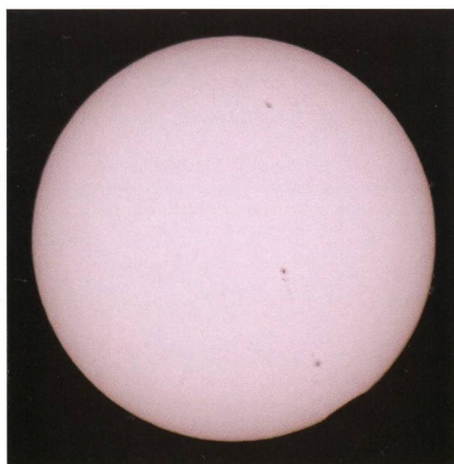
Abbildung 1: Nur wenige Sekunden nach dem ersten Kontakt kann man den Mond bereits als kleine Delle am Sonnenrand erkennen. Dazu muss man den Positionswinkel wissen.
