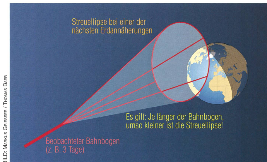
Abbildung 3: Zur Ermittlung von Impakt-Risiken wird der eben bestimmte Bahnbogen eines erdnahen Asteroiden in die Zukunft verlängert, wobei die möglichen Abweichungen berücksichtigt werden. Es entsteht so eine Streuellipse, die bei einem nur kurzen Bahnbogen deutlich grösser ist, als wenn eine längere und entsprechend auch genauere Bahn vorliegt. Mit mathematischen Modellen suchen nun die Bahnspezialisten von Sentry und NEODyS unabhängig voneinander nach Situationen, in denen diese Streuellipse mit unserer Erdkugel eine Deckung hat, wobei in der Regel ein Zeithorizont bis maximal 100 Jahre untersucht wird.
