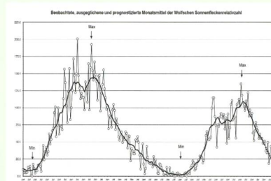
Beobachtete, ausgeglichene und prognostizierte Monatsmittel der WOLFSCHEI Sonnenfleckenzahl
