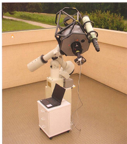
Abbildung 2: Über Jahre hinweg war der 40 cm / f5.9-Hypergraph auf einer älteren Alt-Montierung das Arbeitspferd in der Sternwarte Eschenberg.
