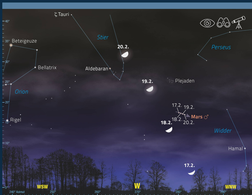
Abbildung 1: Mars ist derzeit der einzige Planet, den man von Auge beobachten kann. Wir sehen hier den Anblick vom 17. bis 20. Februar 2021 gegen 23:30 Uhr MEZ.
