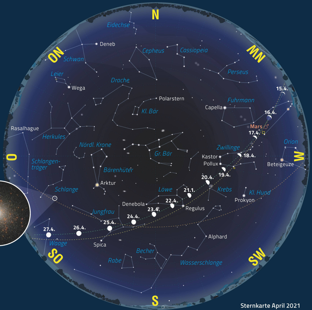
Abbildung 10: Die Planetenpositionen gelten am 15. April 2021.
