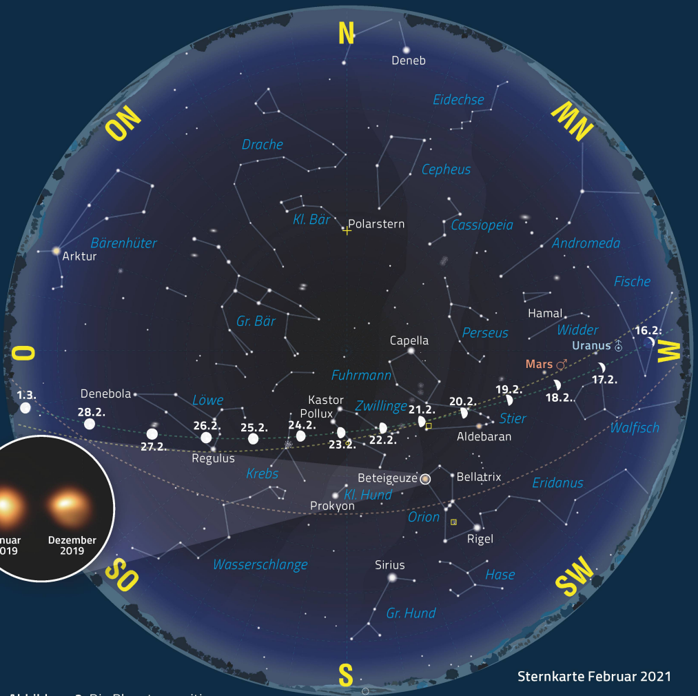
Abbildung 2: Die Planetenpositionen gelten am 15. Februar 2021.
