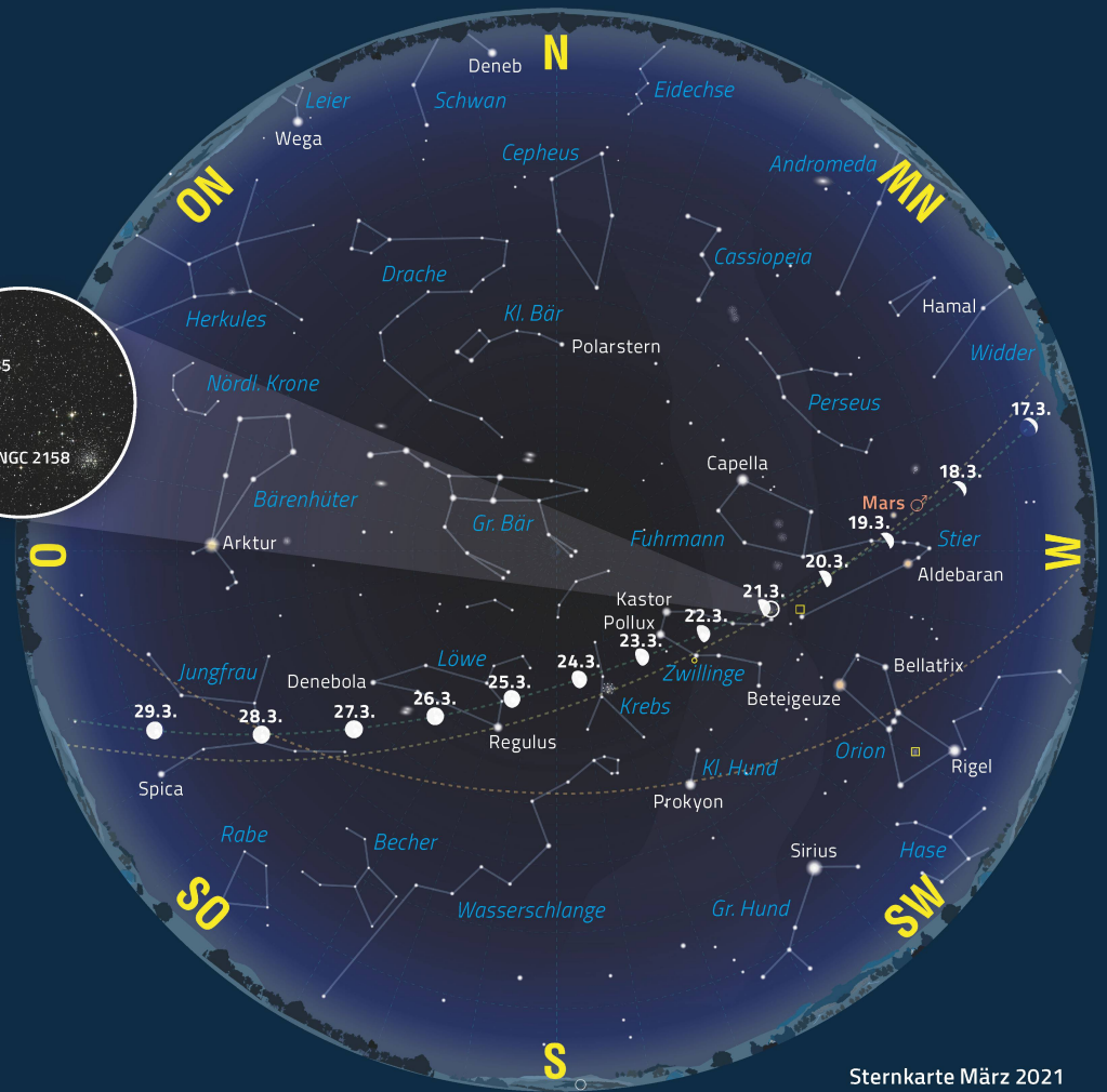
Abbildung 6: Die Planetenpositionen gelten am 15. März 2021.
