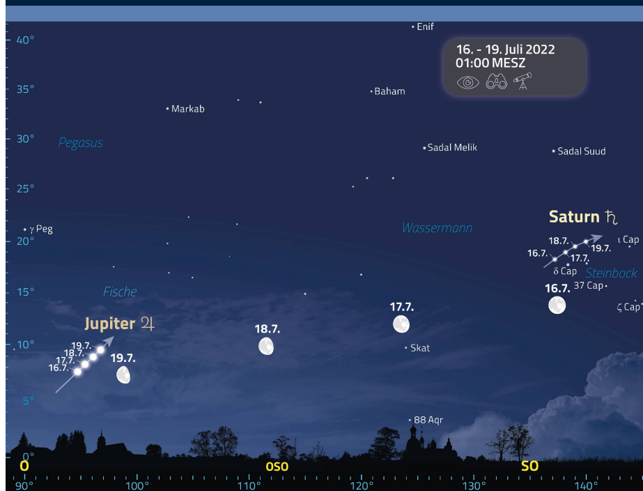
Abbildung 12: Jupiter und Saturn sind nach Mitternacht gemeinsam im Osten und Südosten zu beobachten. Am 16. Juli steht der noch fast volle Mond 4\frac{3}{4}^\circ südlich des Ringplaneten, drei Tage später 3^\circ südlich von Jupiter.
