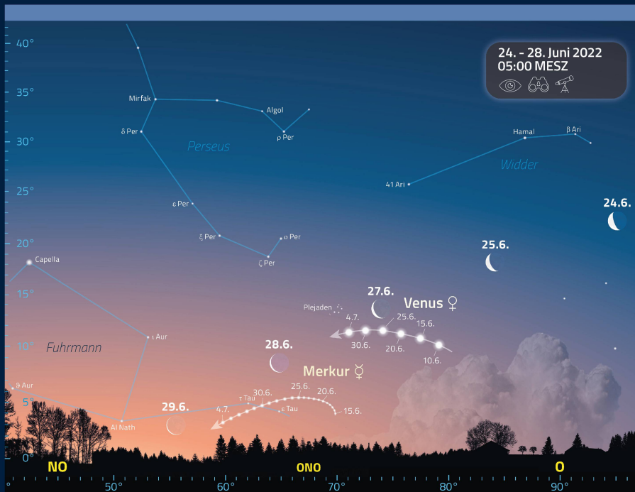
Abbildung 7: Merkur und Venus sind im Juni 2022 gemeinsam am Morgenhimmel zu sehen. Der sonnennächste Planet legt bis zum Monatsende deutlich an Helligkeit zu und kann besonders gut zwischen dem 25. und 30. gesehen werden.
