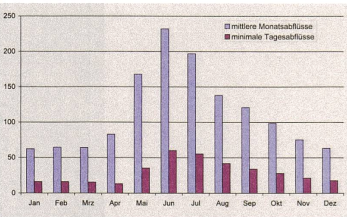
Abb. 1 Abflussmengen im Rhein bei Domat/Ems (Messdaten des BAFU 1962-2006).
