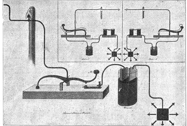
Taf. 2. Telegraph, Tasterapparat.
