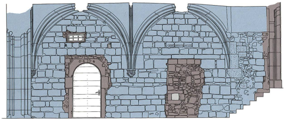
face sud travée 28 travée 29
