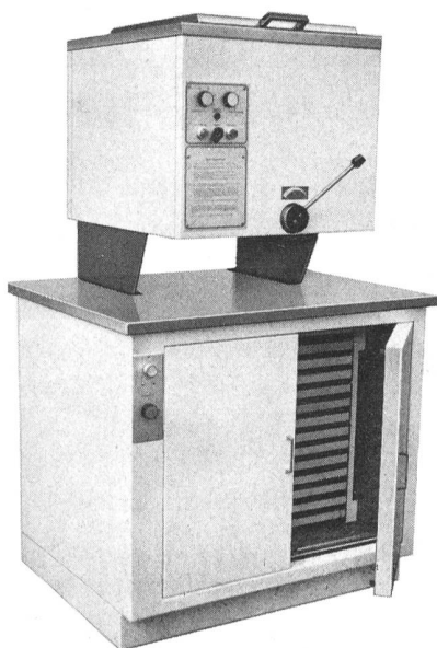
Ruhrwerk TA 60 auf Warmhalteschrank 5070
