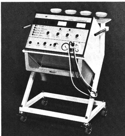
DOELKER PHYSIODYN-DIGITAL Interferenz-Therapiegerät mit Vakuumteil
