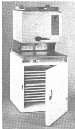
60 Lt. Fangoaufsetzgerät mit Auslauf montiert auf Fangowarm- halteschrank Typ 60. Dazwi- schen Querstromgebläse zur Küh- lung der Fangopackungen.
