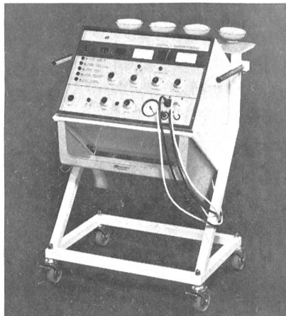
DOELKER PHYSIODYN-DIGITAL Interferenz-Therapiegerät mit Vakuumteil
