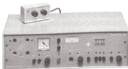
NEMECTRODYN 7 mit Reizzeitgeber S 4000
