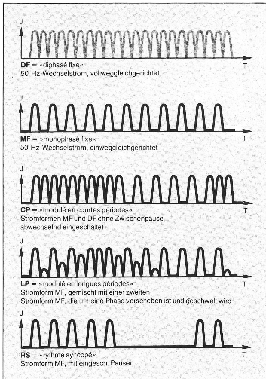
Abbildung 2: Diadynamische Stromformen.
