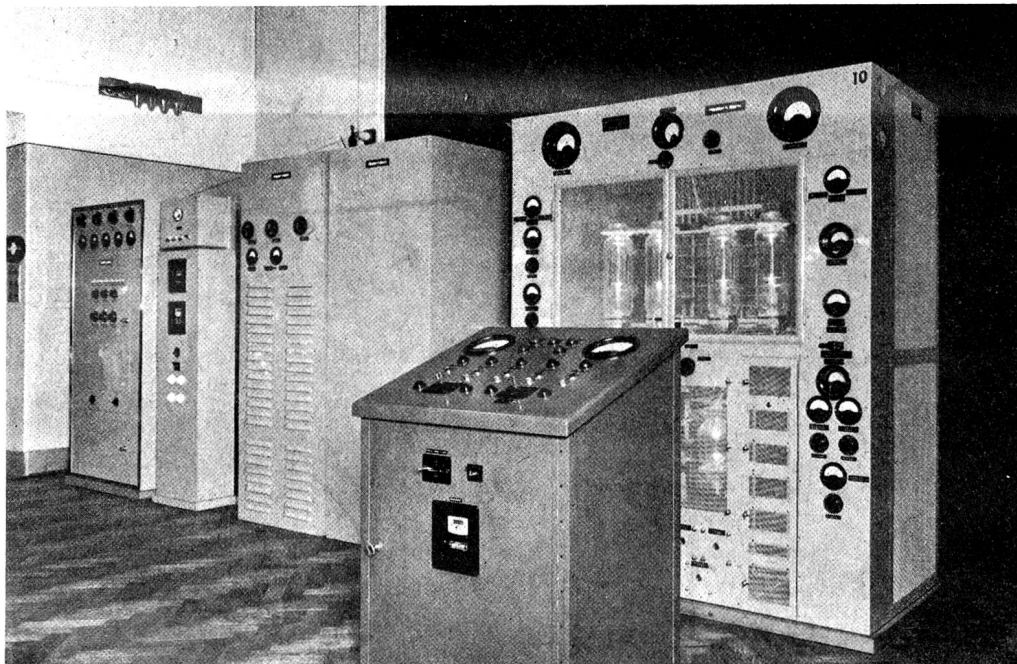
Das Bild zeigt: links einen Nahzonen-Sender für den zivilen Flugverkehr, rechts einen Kurzwellen-Telegraphie-Sender für den Verkehr mit Übersee
