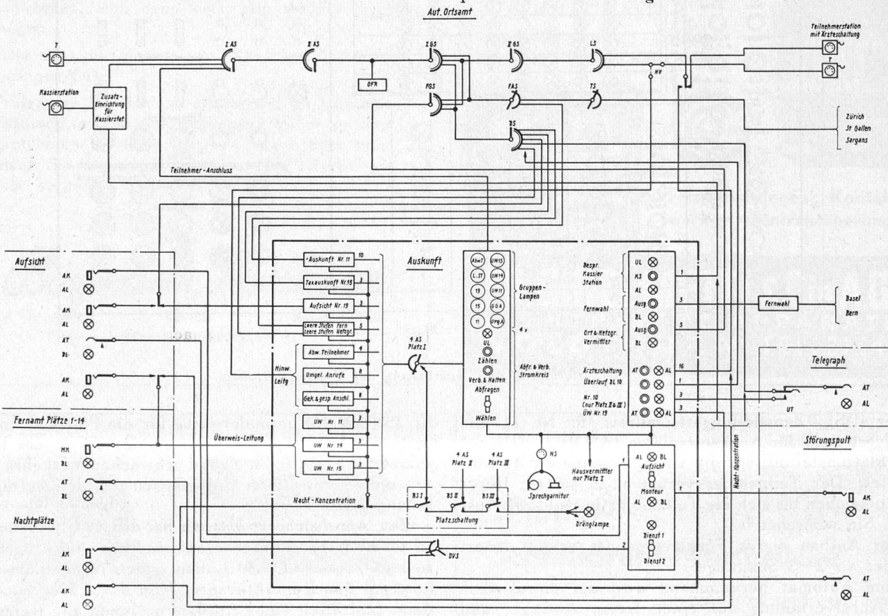
Fig. 3. Verbindungsdiagramm der Auskunft Chur.
