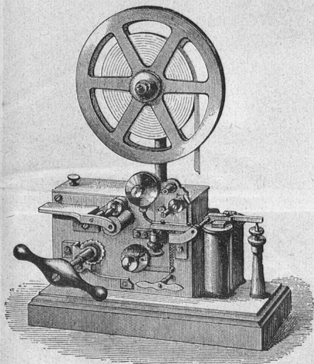
Alter Morse-Farbschreiber
