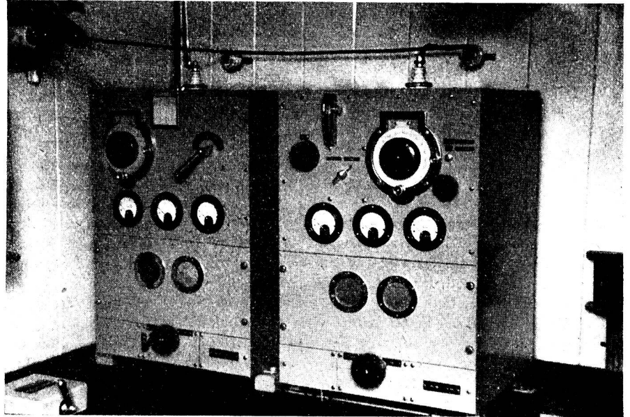
Lang- und Kurzwelligensender auf der „Albula“
