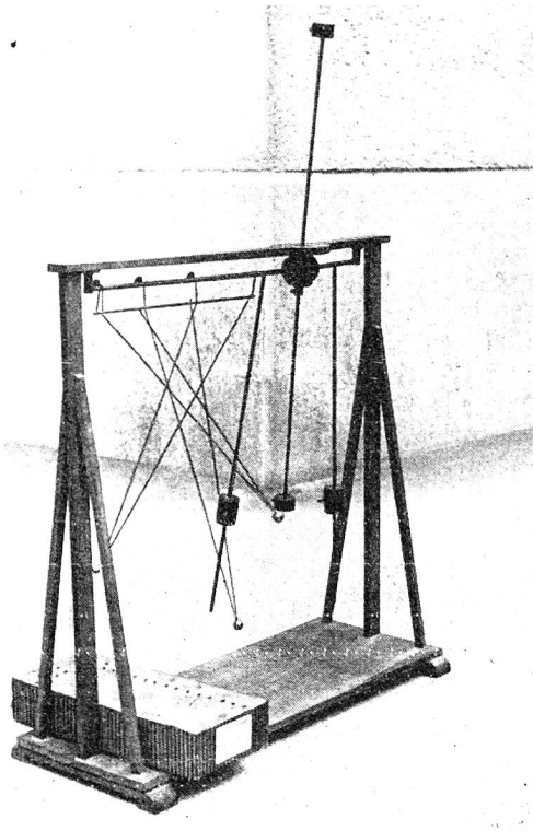
Seitliche Momentaufnahme der Kopplungsschwingungen . (Aeussere Fadenpendel in Schwingung. Mittleres Fadenpendel in Ruhe.) Phot. Hans Meiner, Zürich.
