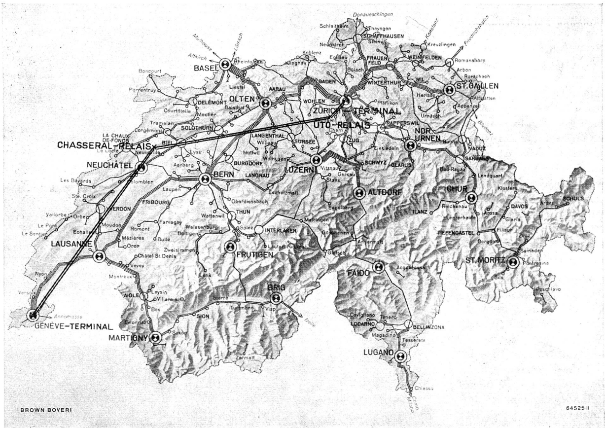
Das schweizerische Telephonkabelnetz mit eingezeichneter Mehrkanal-Richtstrahlanlage Zürich—Genf
