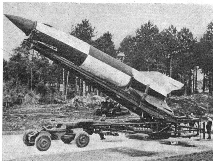
Schussbereitmachen der V-2
