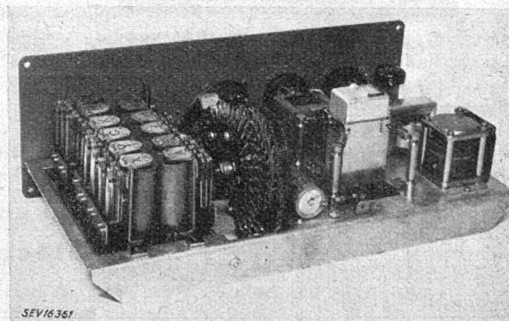
Fig. 4 Anruf- und Steueraggregat
