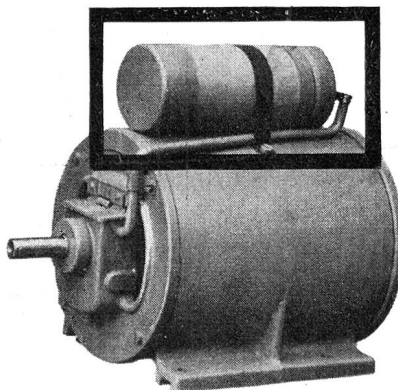
Condensateur de démarrage STANDARD monté sur moteur Condex-Oerlikon
