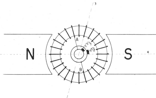
Fig. 142 1 et 2 Bornes 3 Ligne neutre 4 Ligne des pôles
