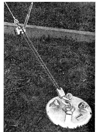
«Terrax / Erdix» Bodenanker aus Stahl, 2–6 t. Für temporäre Verankerungen auch in schwerem Boden.
