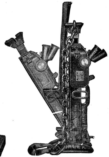
«Simplex»-Universalwinden mit Gelenkfuss: 522 310A 2030 Kapazität in t: 5 15 20 Hub in mm: 355 355 480 Mit 2 Standard- und 1 bzw. 2 Spezialzubehören lieferbar.
