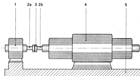
Fig. 147 1 l'excitatrice 3 Couplage (fixe) 2 a l'arbre de l'excitatrice 4 Alternateur 2 b l'arbre de l'alternateur 5 Plaque de base
