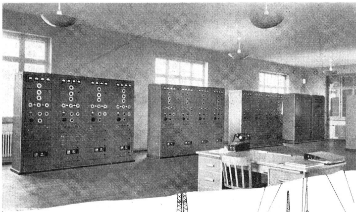
Brown Boveri Sender für den Flugsicherungsdienst in der Sendestation Walthikon bei Zürich
