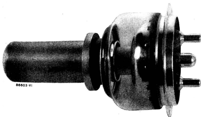
Eine typische Vertreterin aus der Reihe der Brown Boveri Kurzwellen-Sendetrioden mit thorierter Kathode, die Triode BTL (BTW) t-1 für forcierte Luft- (BTL) oder Wasserkühlung (BTW). Ihre Anodenverlustleistung beträgt 6 (10) kW.
