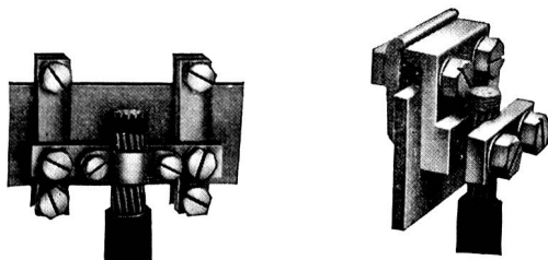
Klemmen für Flachkupferschienen
