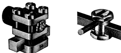
Sammelschienenkasten aus Blech und Guss
