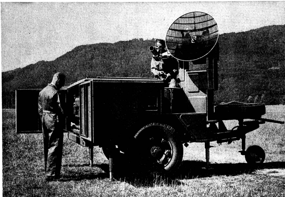
ALBIS-Feuerleitradar AFR 406
