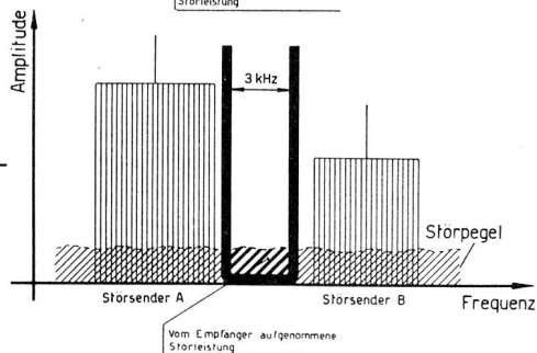
Fig. 9. Empfänger-Selektivität mit zwei Störsendern.
