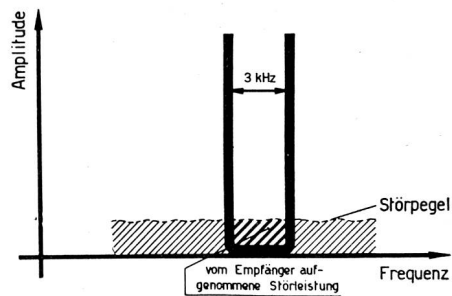
Fig. 8. Empfänger-Selektivität.
