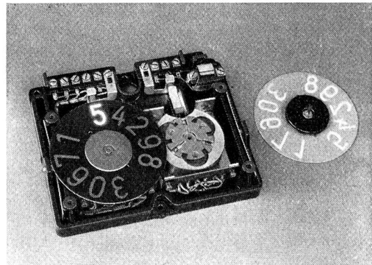
Nummernanzeigesystem in Personensuch-Tableau, ohne Verschaltung
