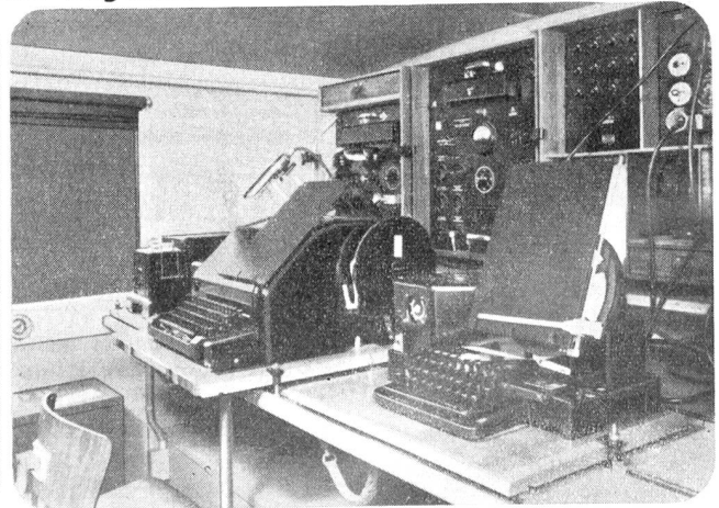
Fernschreibstation mit automatischem Sender und Lochstreifenstanzer für Doppelstrom- oder Eintönübertragung.
