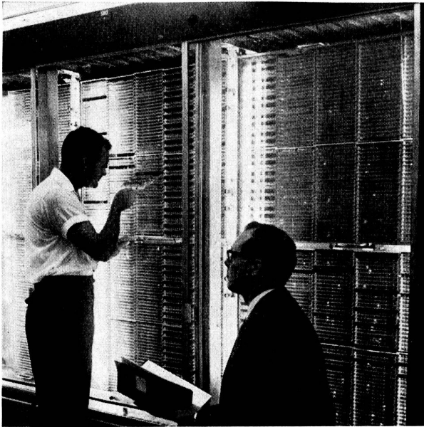
Teilansicht des elektronischen Telephonamtes in Morris (USA). Über die in den Gestellen reihenweise angeordneten Kaltkathodenröhren werden die Sprechwege durchgeschaltet. Die Lichtpunkte im rechten Gestell weisen auf gezündete Röhren, also auf durchgeschaltete Verbindungen, hin.
