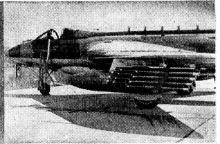
auf HUNTER-Flugzeug
