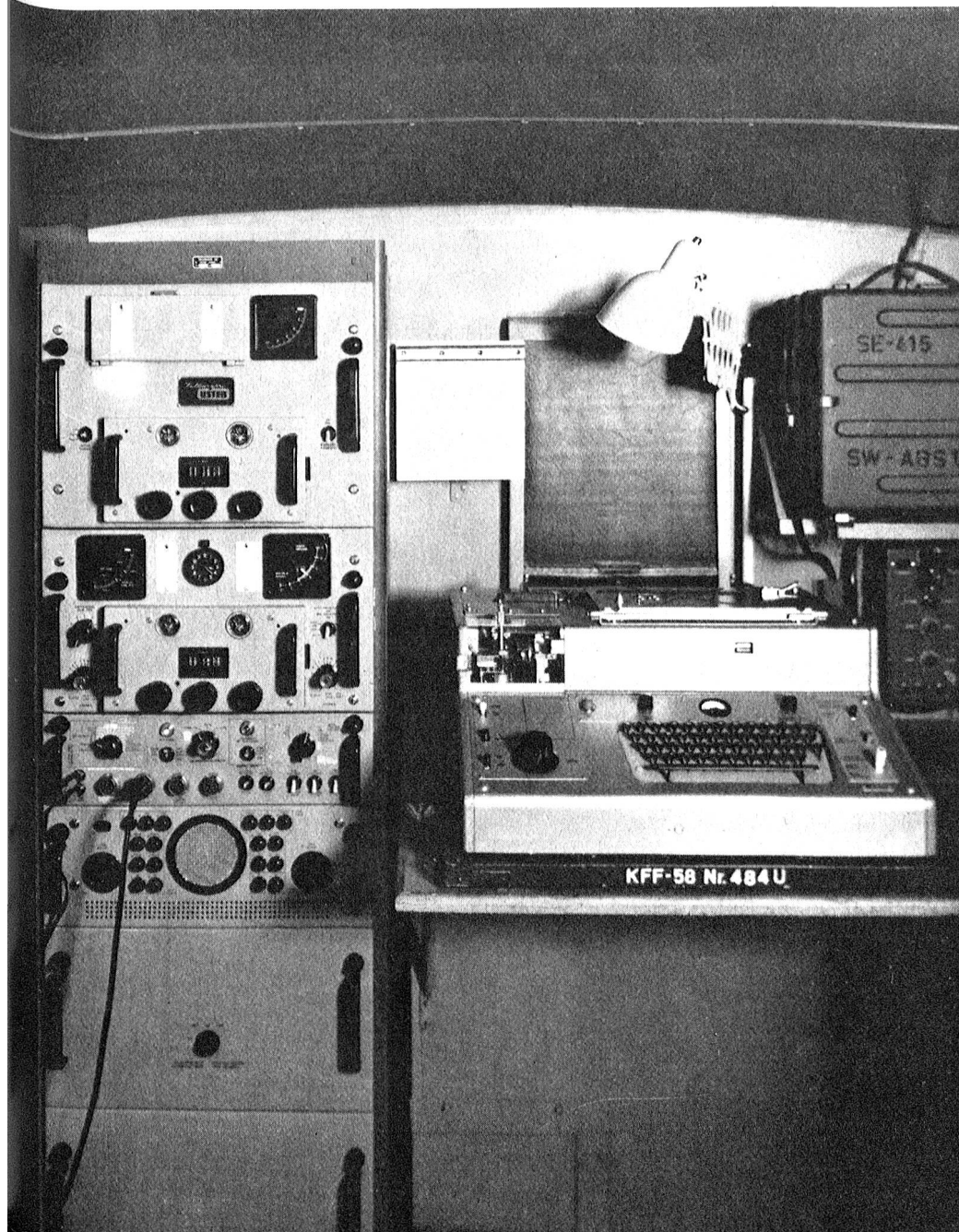
Innenansicht der neuen 1-kW-Grossfunkstation SE-415
