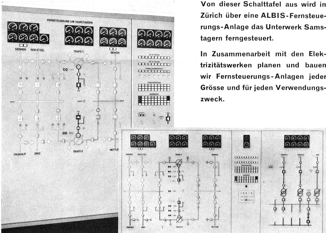
Fernsteuer - Schalttafel Zürich - Binz
