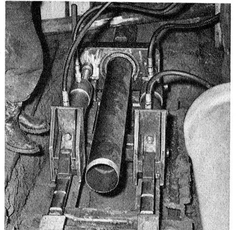
Röhrenstosspressen mech. und hydr.
