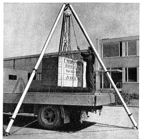
Dreibeine HERCULES
