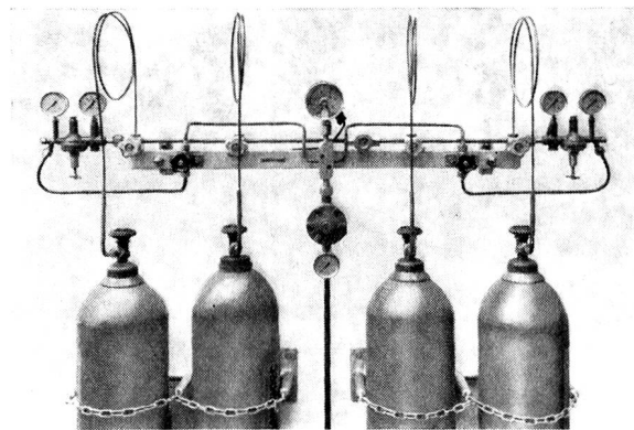
Stationäre Sauerstoff-Versorgungs-Zentrale
