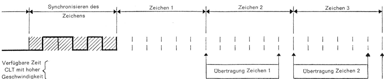
Fig. 14. Synchroner Datenübertragung (6 Kanal)
