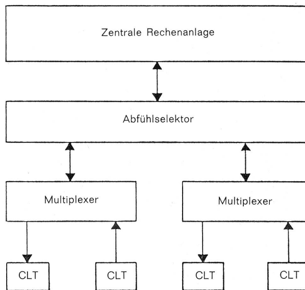
Abbildung 11: Mehrere Multiplexer pro E/A-Kanal mit einem Abfühlsektor.
