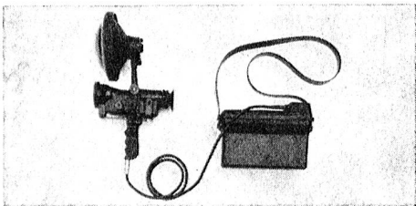
ALBIS-IR-Beobachtungsgerät «ARGUS»
