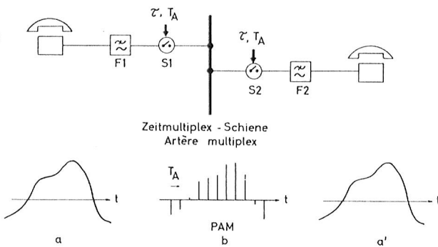
Fig. 4: Sprechweg durch ein Zeitmultiplex-Koppelnetzwerk
