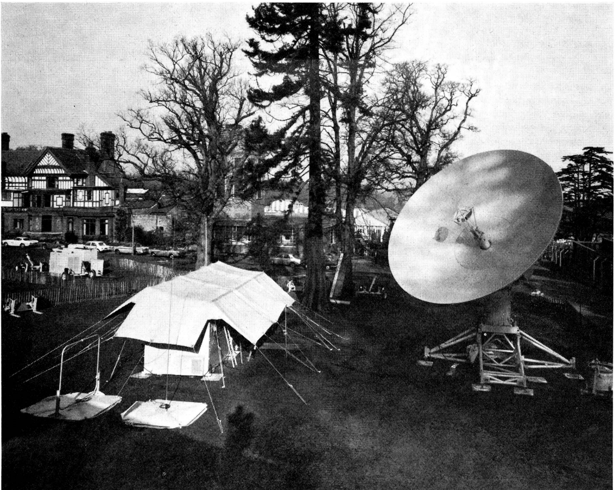
Eine mobile Bodenstation des Typs 4 für das britische Fernmeldesatellitensystem Skynet, hergestellt von der GEC/AEI (Electronics) Limited. Die ganze Station lässt sich in je rund 1800 kg schwere Einheiten zerlegen, in zwei Lockheed C-130 Hercules transportieren und in vier Stunden von sechs
